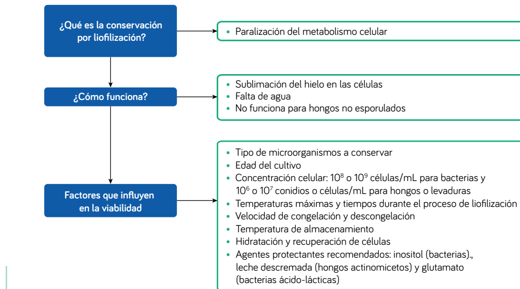
Figura 3. Características de la conservación por liofilización.
