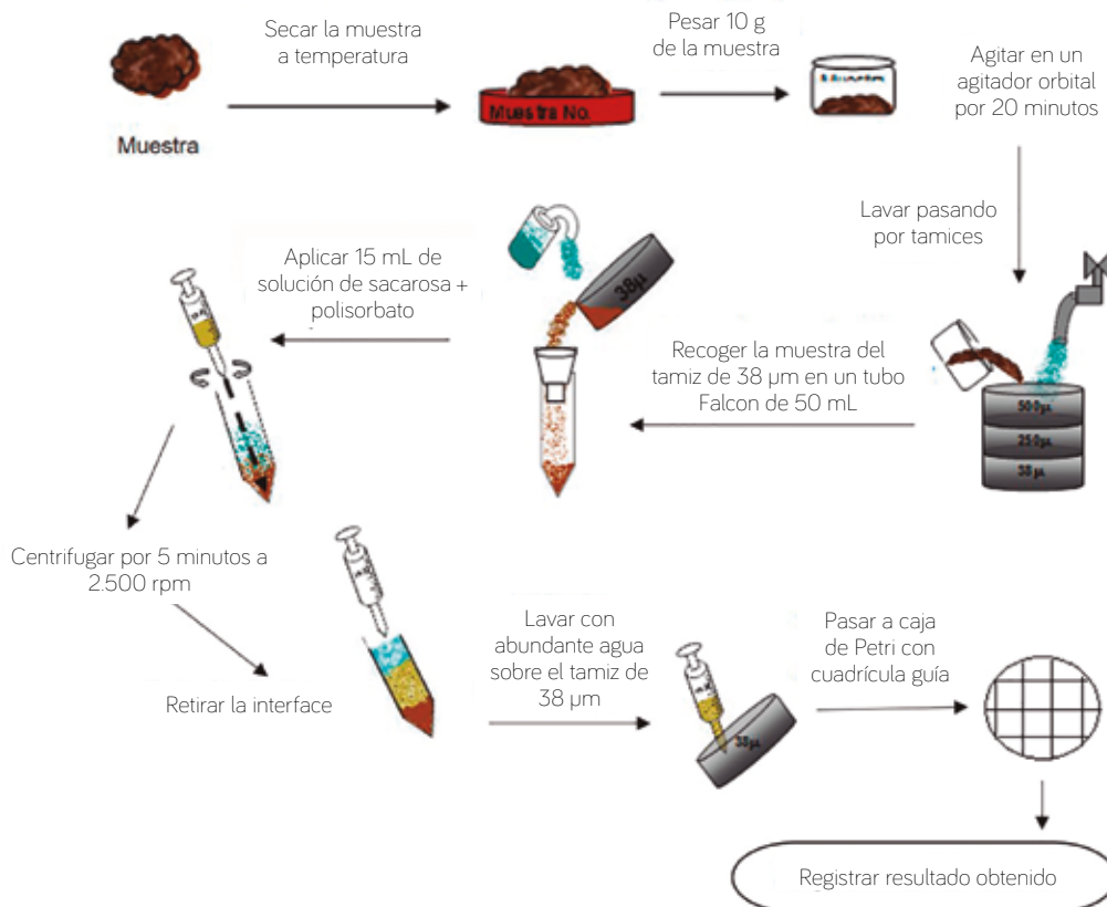
Figura 12. Método para el aislamiento de esporas de HFMA a partir de muestras de suelo.
