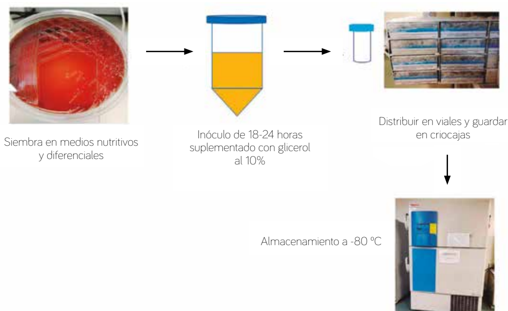
Figura 57. Flujo de trabajo de crioconservación a -80 °C para bacterias Gram-positivas y Gram-negativas.
