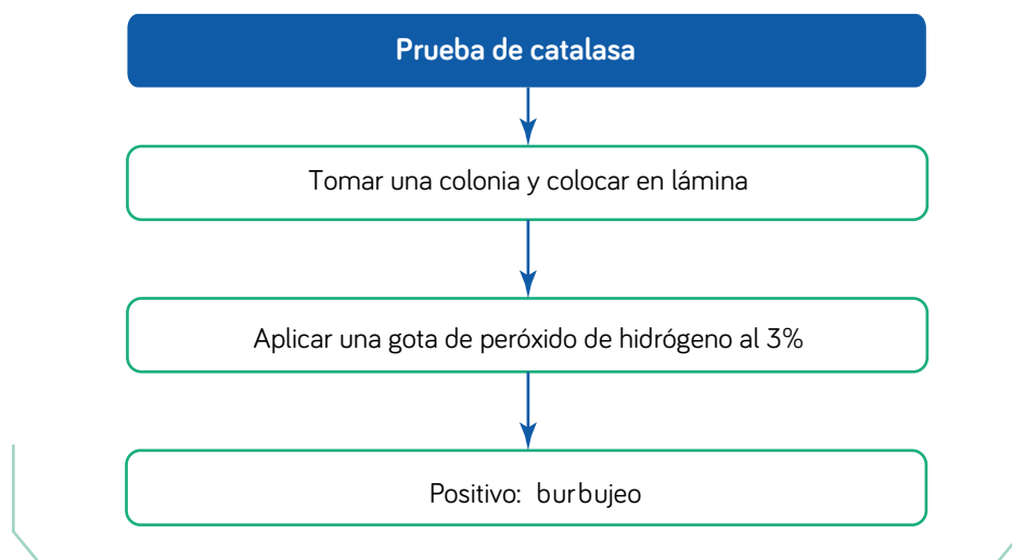
Figura 51. Procedimiento para la prueba de catalasa.
