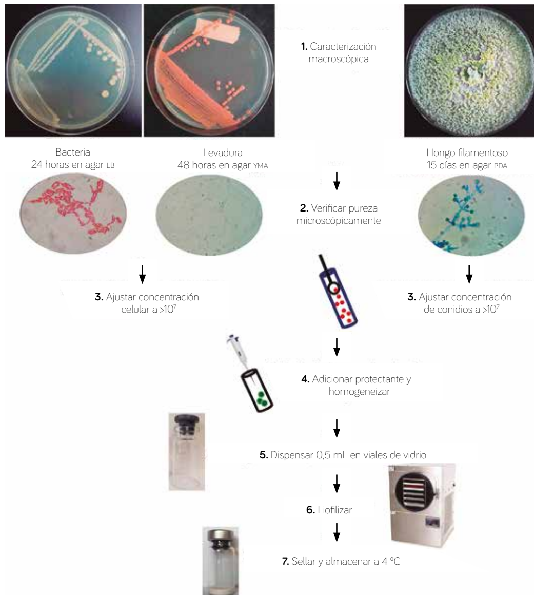
Figura 22. Procedimiento para la conservación de bacterias, levaduras y hongos filamentosos con el método de liofilización.
