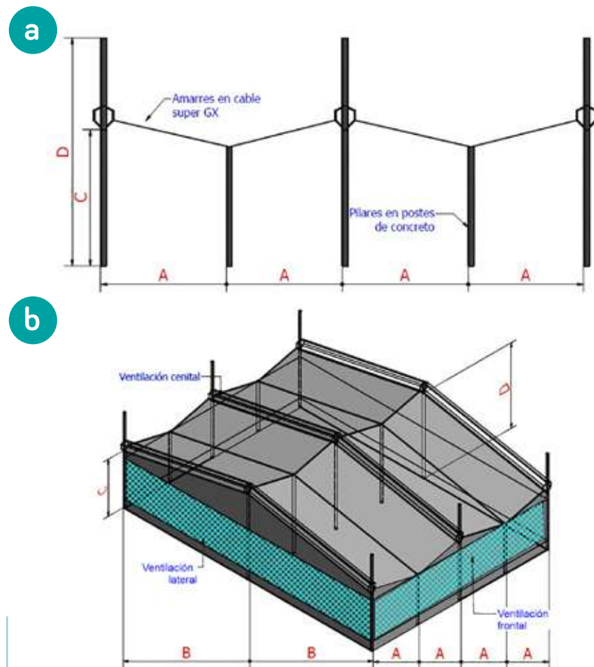
Figura 6. Esquema general del invernadero espacial a. Esquema geométrico del pórtico; b. Arquitectura típica del invernadero espacial.
