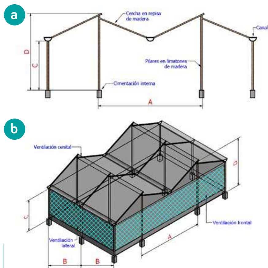
Figura 5. Esquema general del invernadero colgante a. Esquema geométrico del pórtico; b. Arquitectura típica del invernadero colgante.
