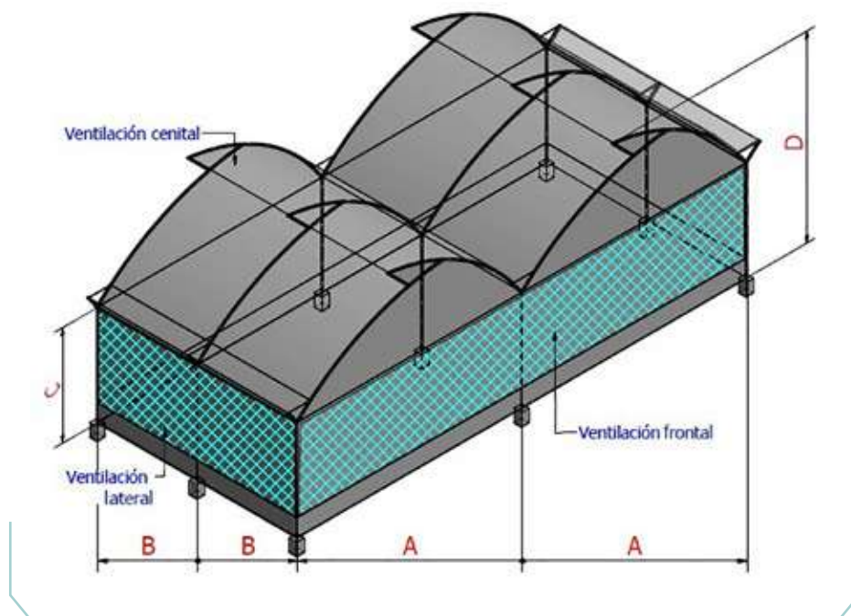
Figura 9. Arquitectura del invernadero tipo túnel con cubierta gótica.
