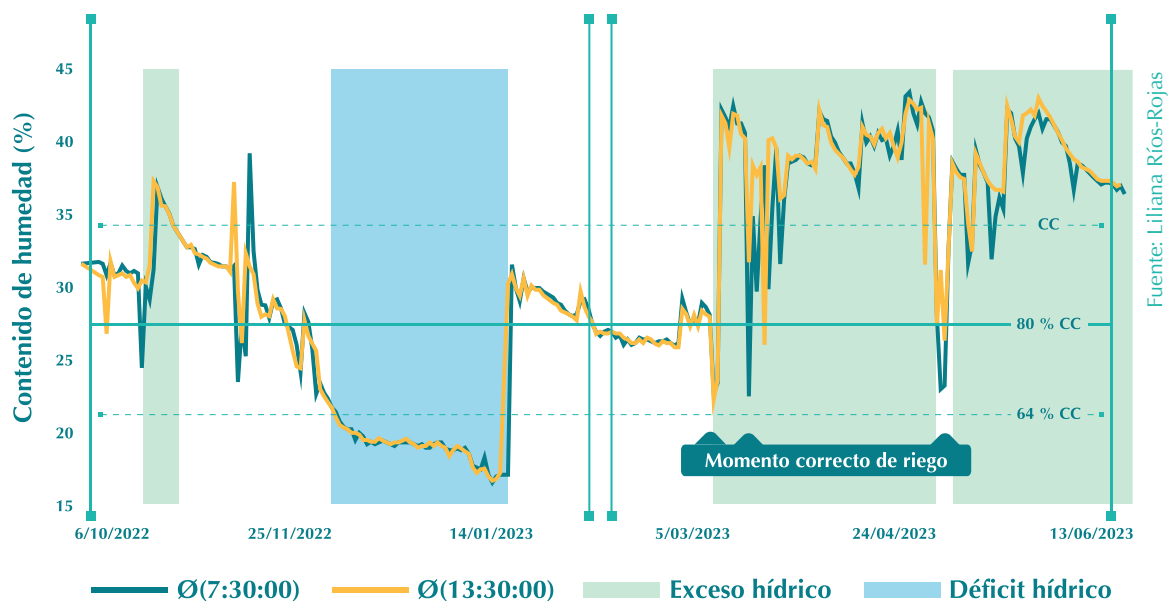
Figura 23. Fracción de una serie de sensor de humedad del suelo.
